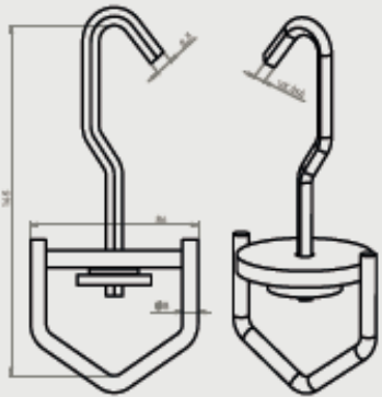
OTOČNÝ SYSTÉM DV.03
