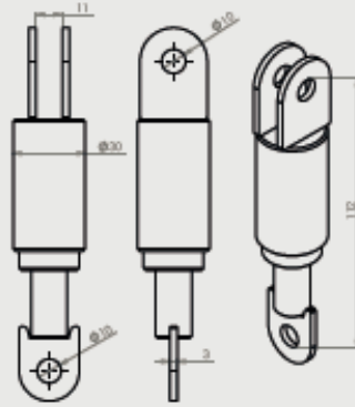
OTOČNÝ SYSTÉM DV.03
